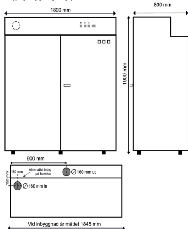
Måttskiss TS 180 E
